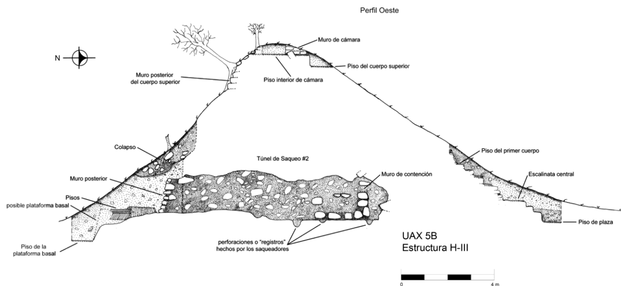
Figura 7 Corte Norte-Sur de la Estructura H-III (Dibujo M. Pellecer, digitalización E. Arredondo) SAHI-Uaxactun 2009.
